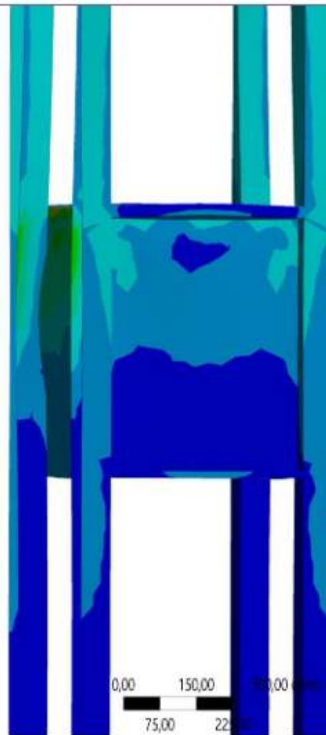
Рисунок 12 – Расчетные результаты напряжений и деформаций противовеса ш. Южнодонбасская №1
