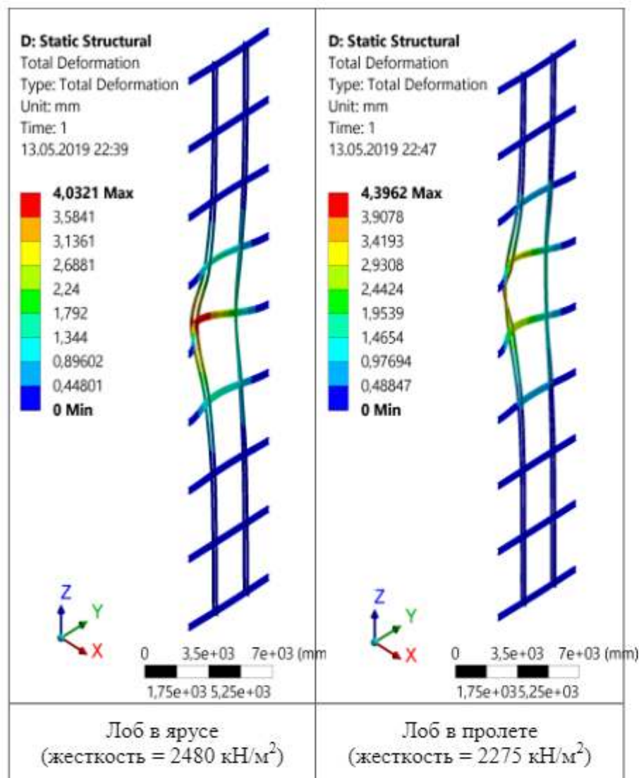
Рисунок 2 – Результаты расчета при лобовом направлении приложенной силы
