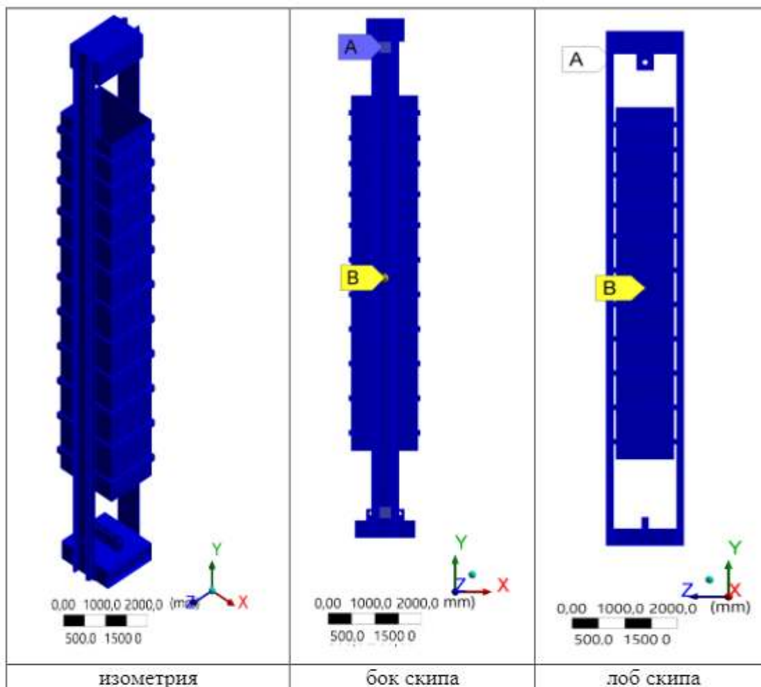
Рисунок 9 – ТТМ скипа CHM 25
