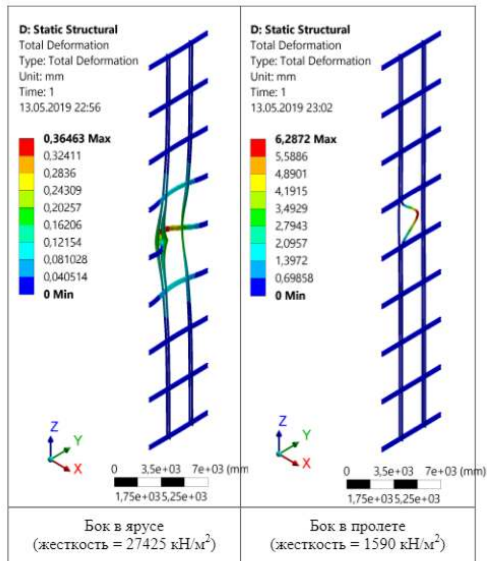
Рисунок 3 – Результаты расчета при боковом направлении приложенной силы
