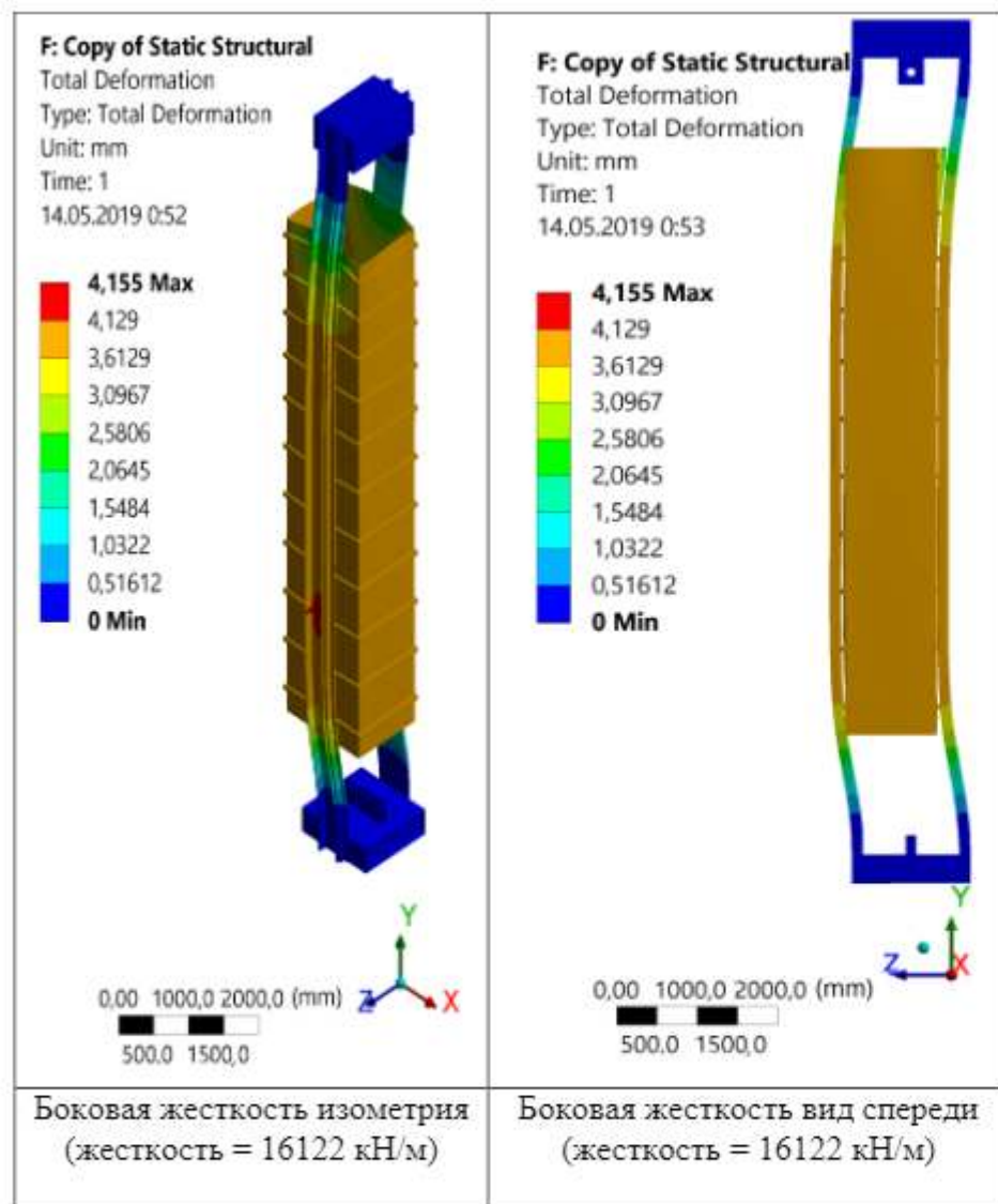
Рисунок 10 – Результаты расчета при боковом направлении приложенной силы Слип CHM 25
