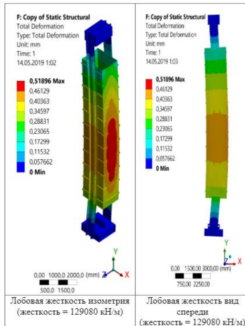
Рисунок 11 – Результаты расчета при лобовом направлении приложенной силы Слип CHM 25
